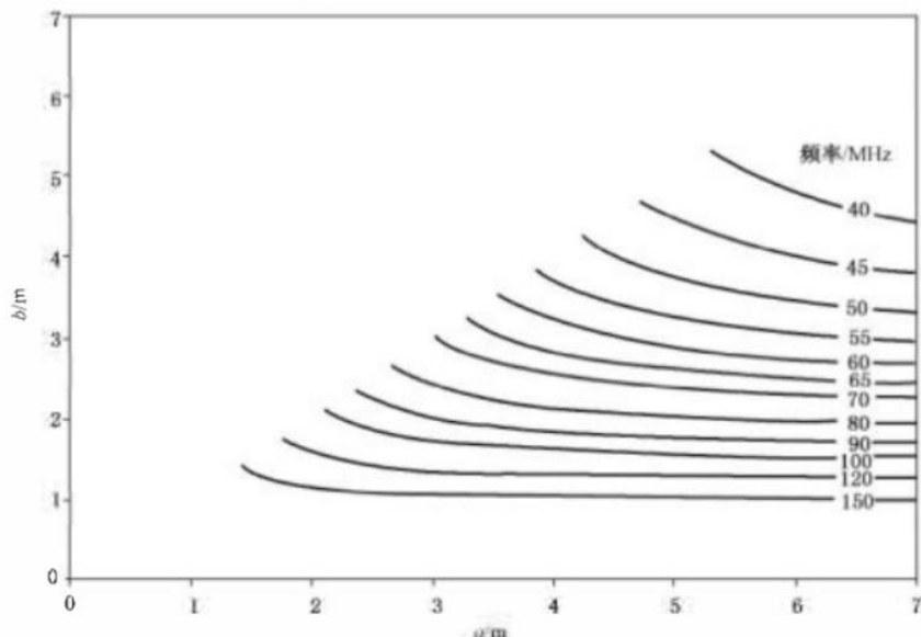
图 5 最低固有谐振频率图
