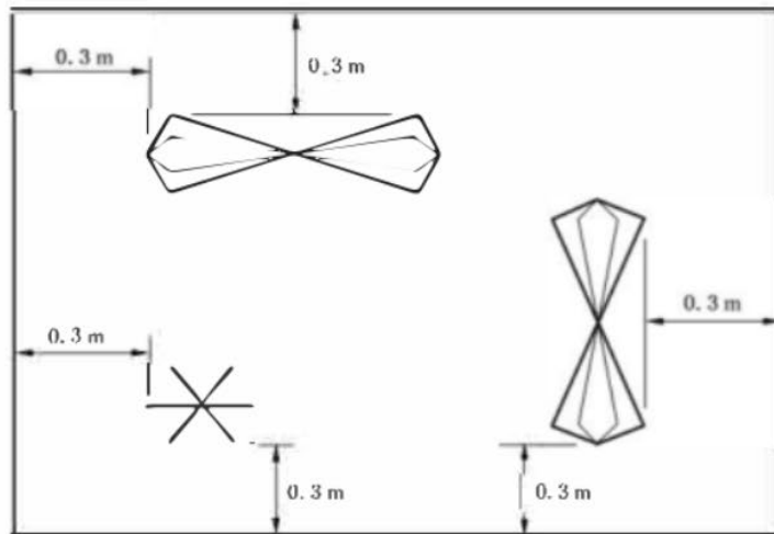
图 E.1 天线到屏蔽壁的最小距离
