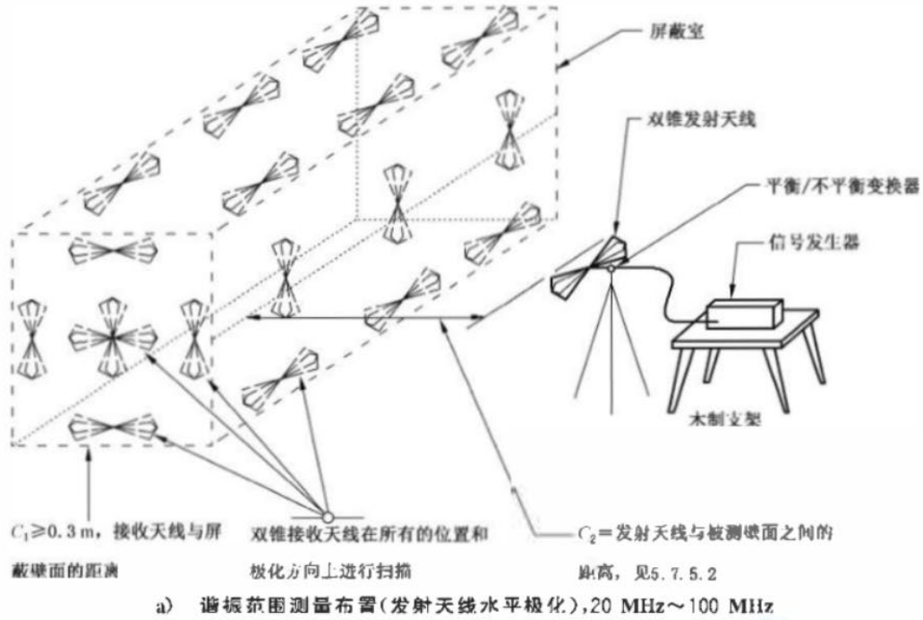
图4 谐振范围测量布置示意图
