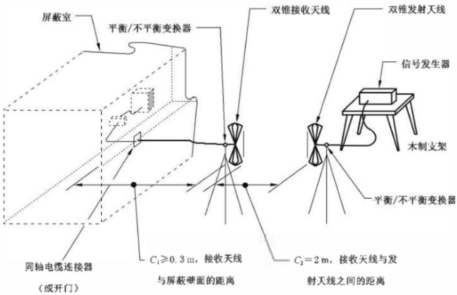
b) 谐振范围参考电平测量布置(垂直极化), 20 MHz~100 MHz
