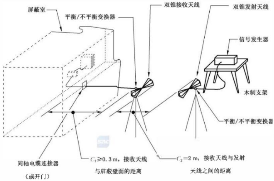
a) 谐振范围参考电平测量布置(水平极化), 20 MHz~100 MHz
