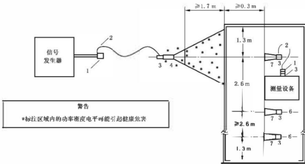
a) SE 测量布置
