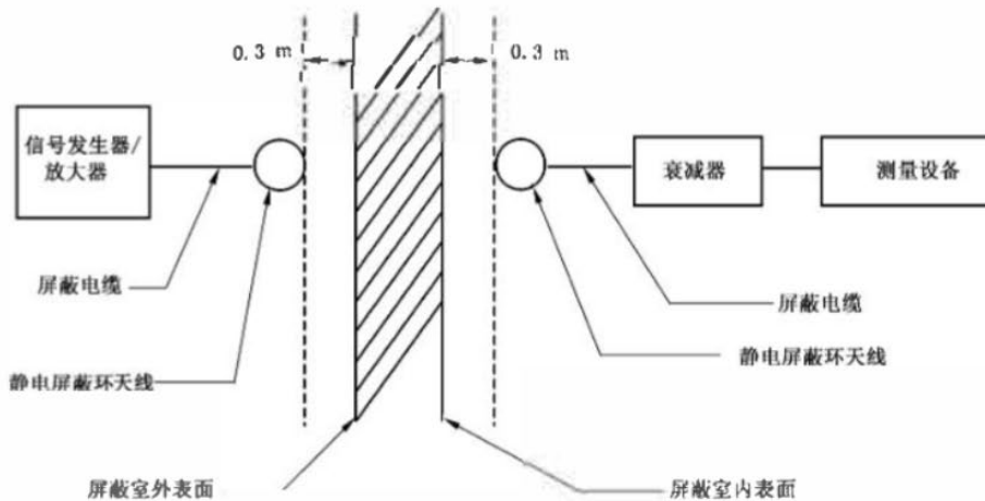
图 1 磁场测量布置
